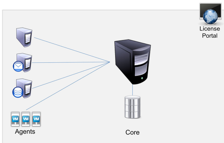
Figure 2. Architecture de déploiement AppAssure 5 de base
