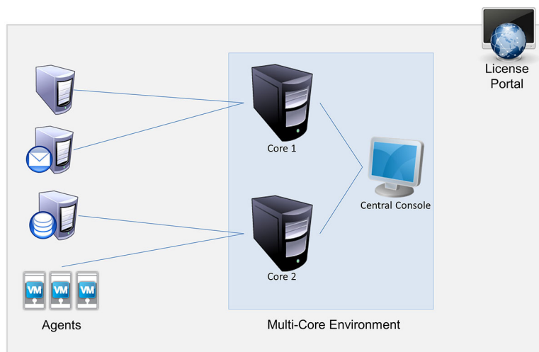
Figure 3. Architecture de déploiement AppAssure 5 avec plusieurs cores
