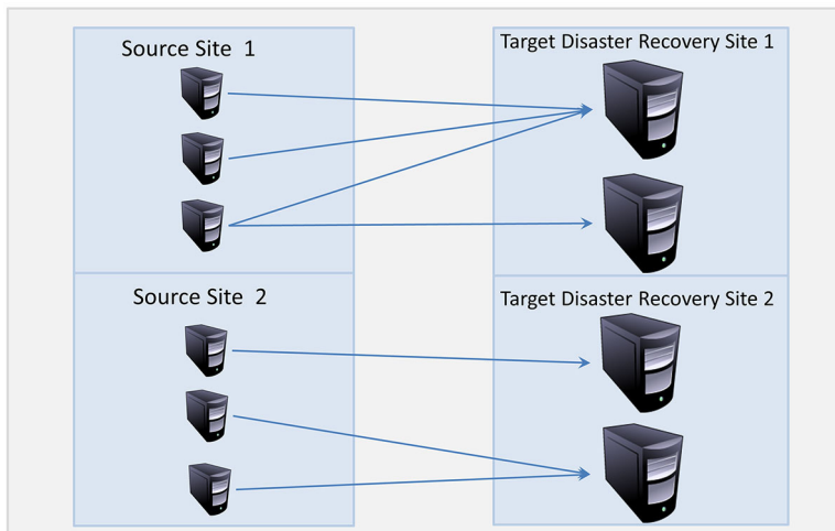
Figure 9. Diagramme de l'architecture de réplication multipoint
